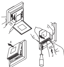
FIG. 3 BR1033A03A2
