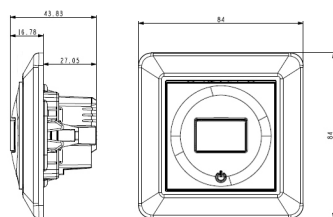
Målskisse
