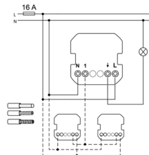
Koblingsskjema
